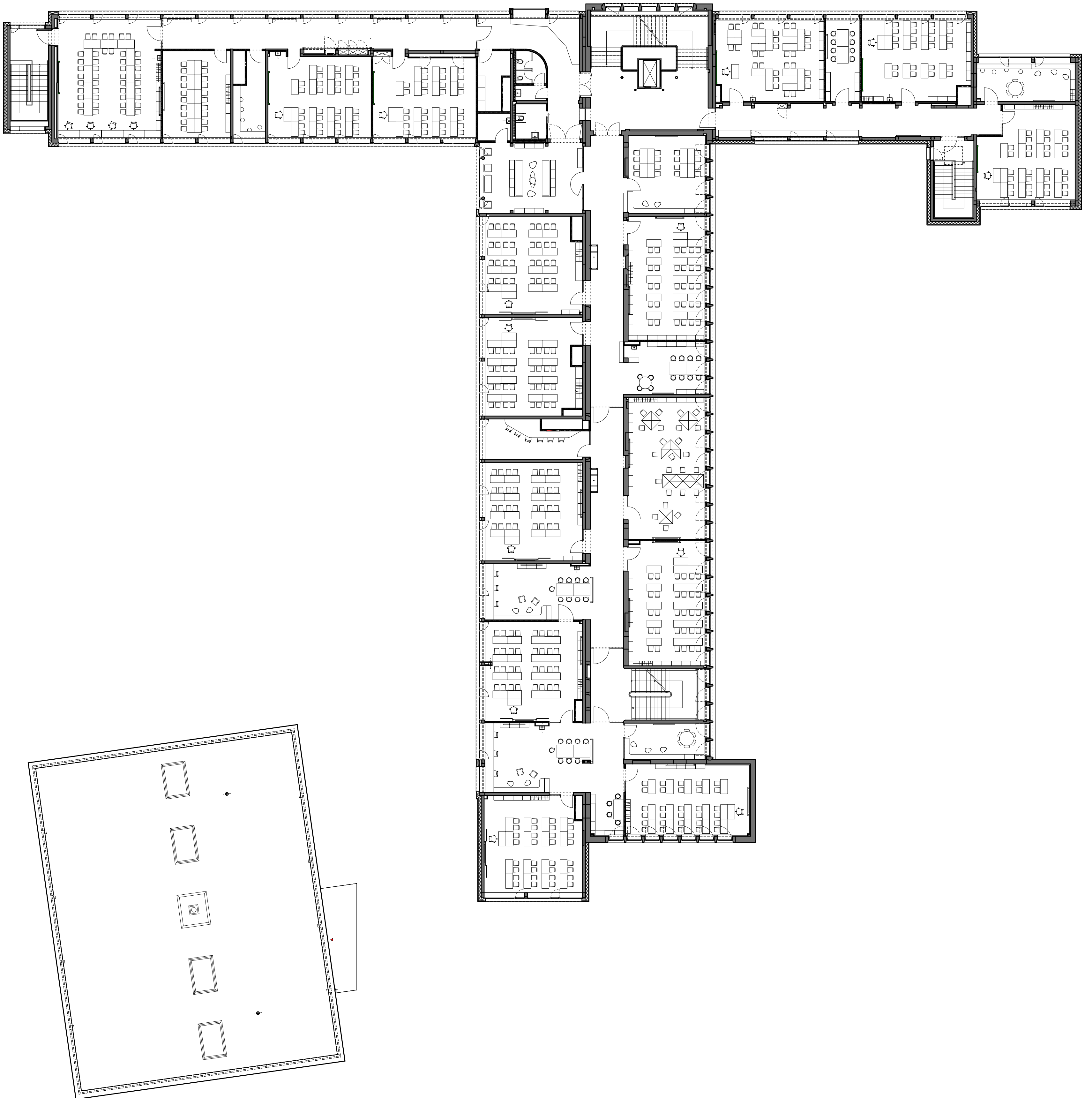
2. OBERGESCHOSS, M1:200
