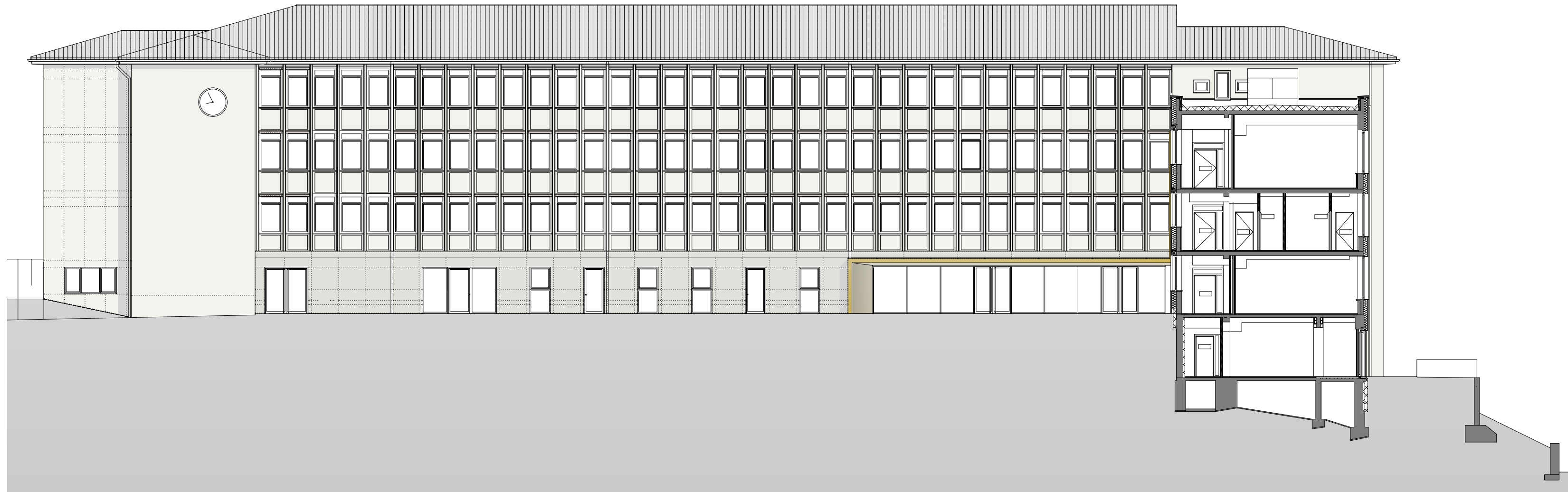
SCHNITTANSICHT OST, M1:200
